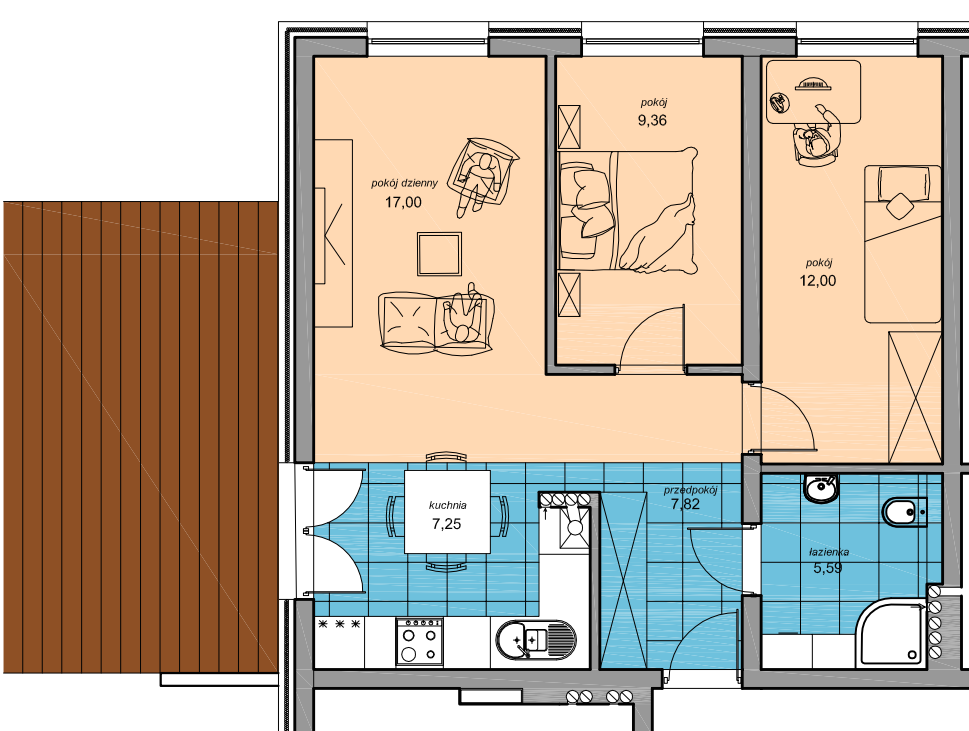
RZUT MIESZKANIA
