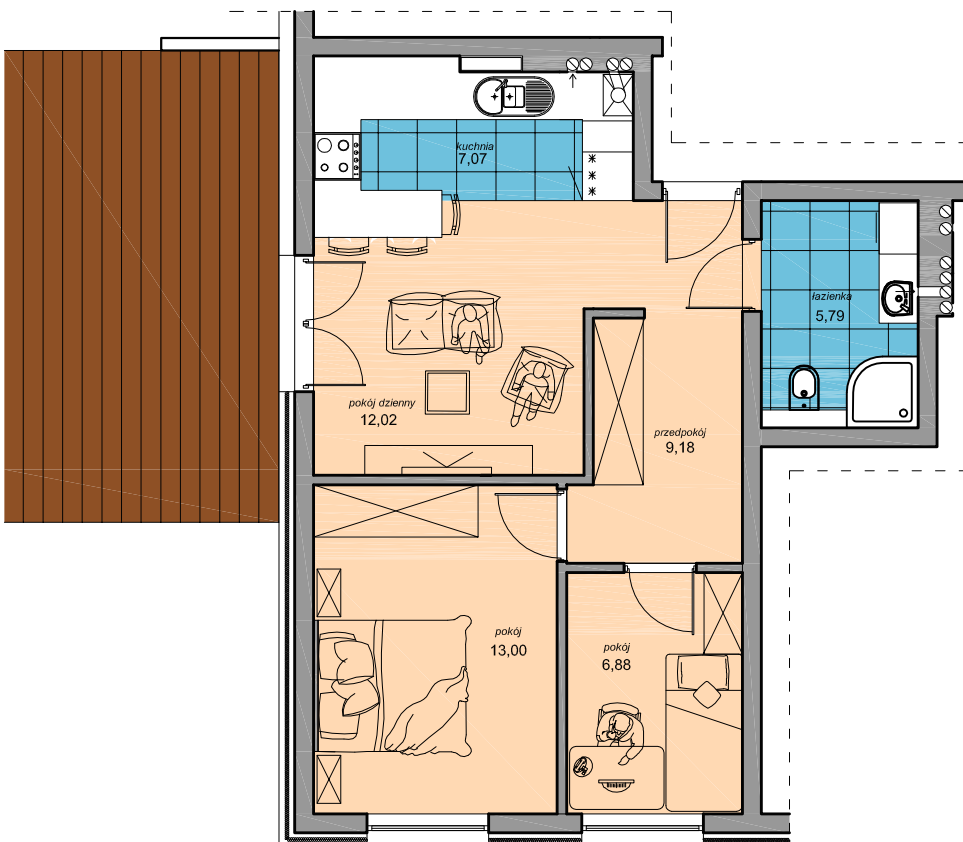
RZUT MIESZKANIA
