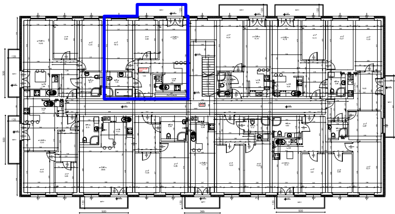
RZUT KONDYGNACJI II II PIĘTRA
