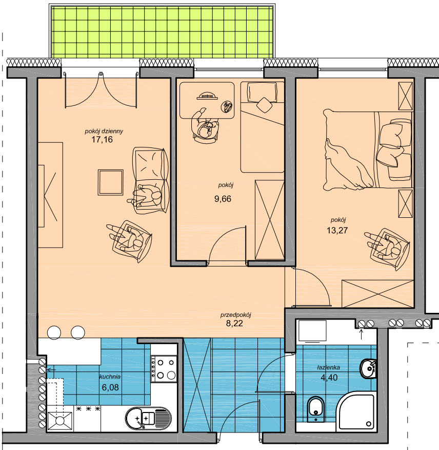
RZUT MIESZKANIA
