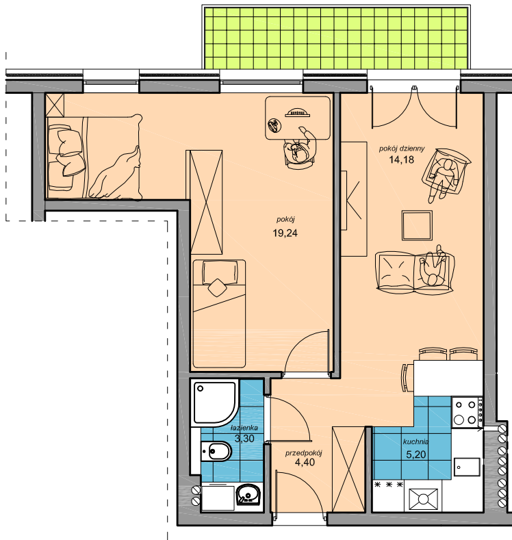
RZUT MIESZKANIA
