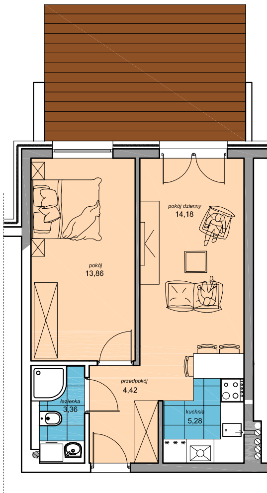
RZUT MIESZKANIA
